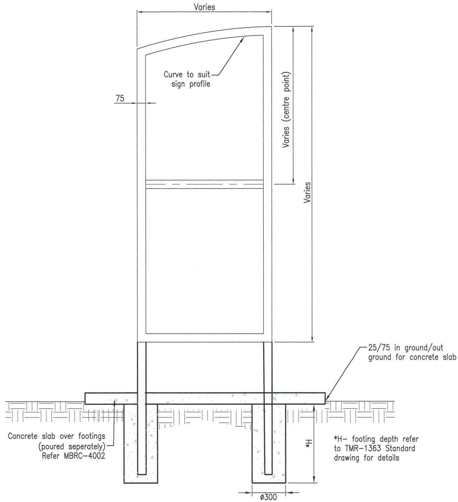
ELEVATION
